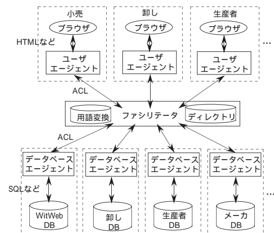
図 1 SAGE:Francis の構成
